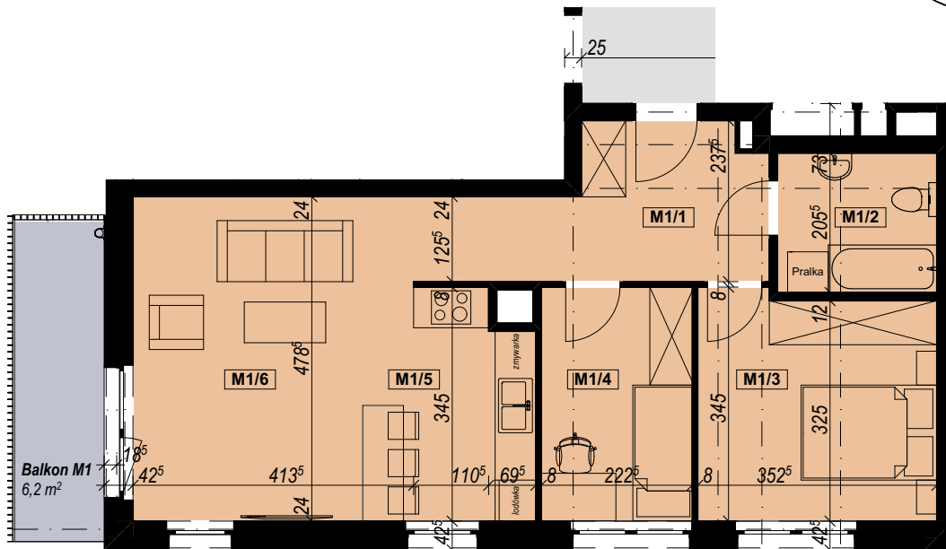
RZUT MIESZKANIA 1:100
