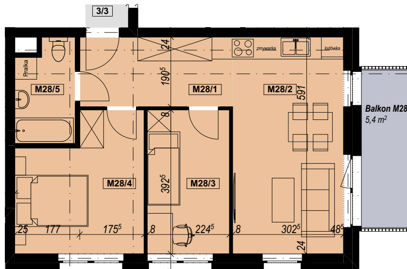
RZUT MIESZKANIA 1:100
