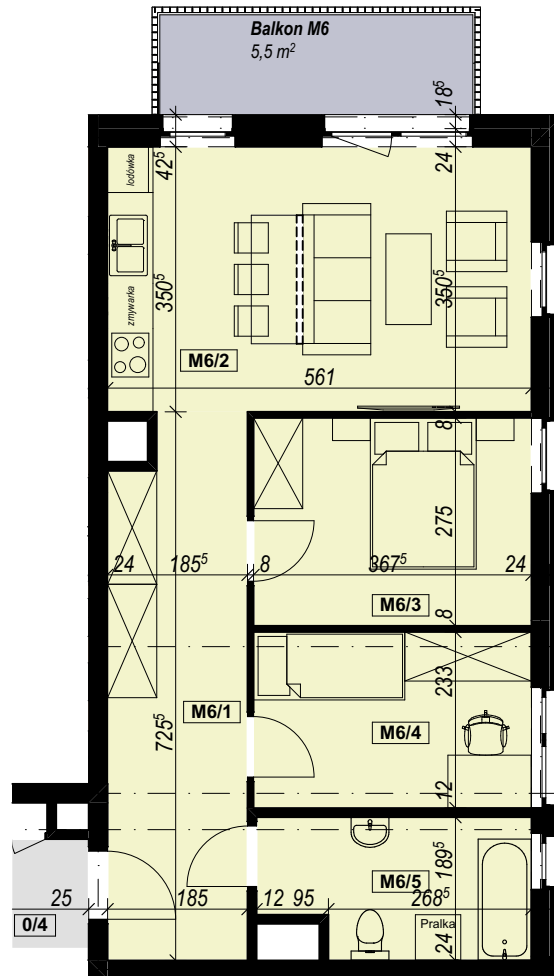
RZUT MIESZKANIA 1:100
